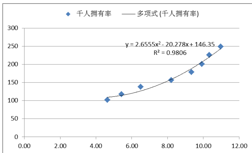
图 4.4 机动车保有量预测模型
